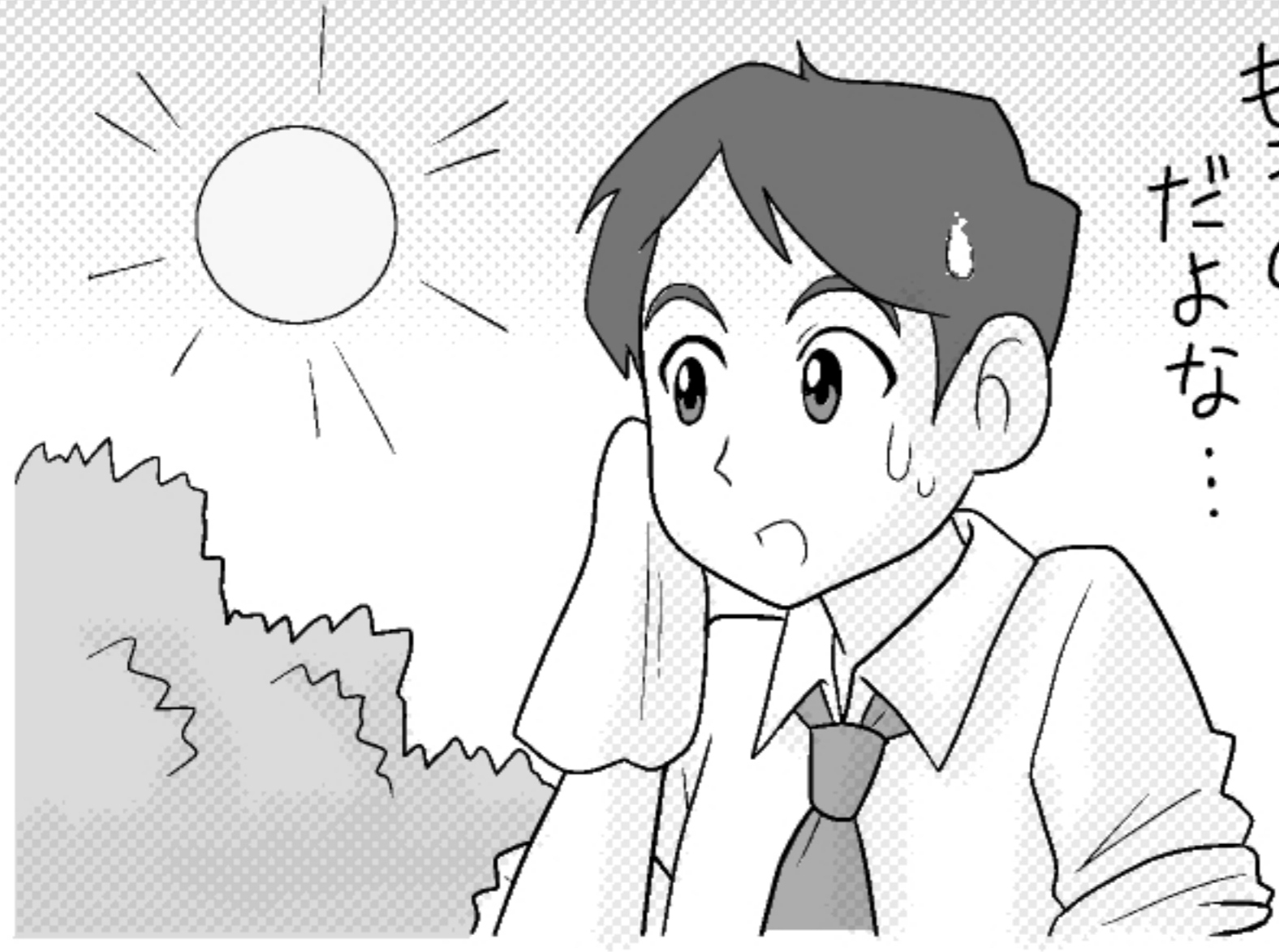
地球の温暖化
