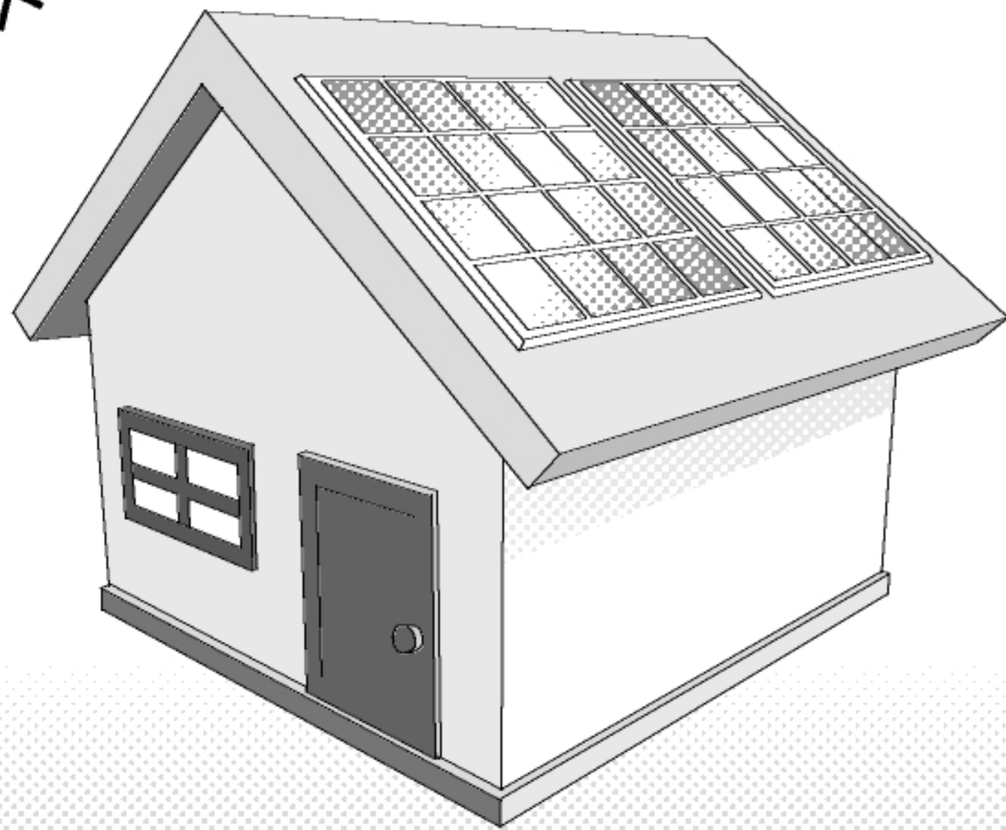
エネルギー問題
